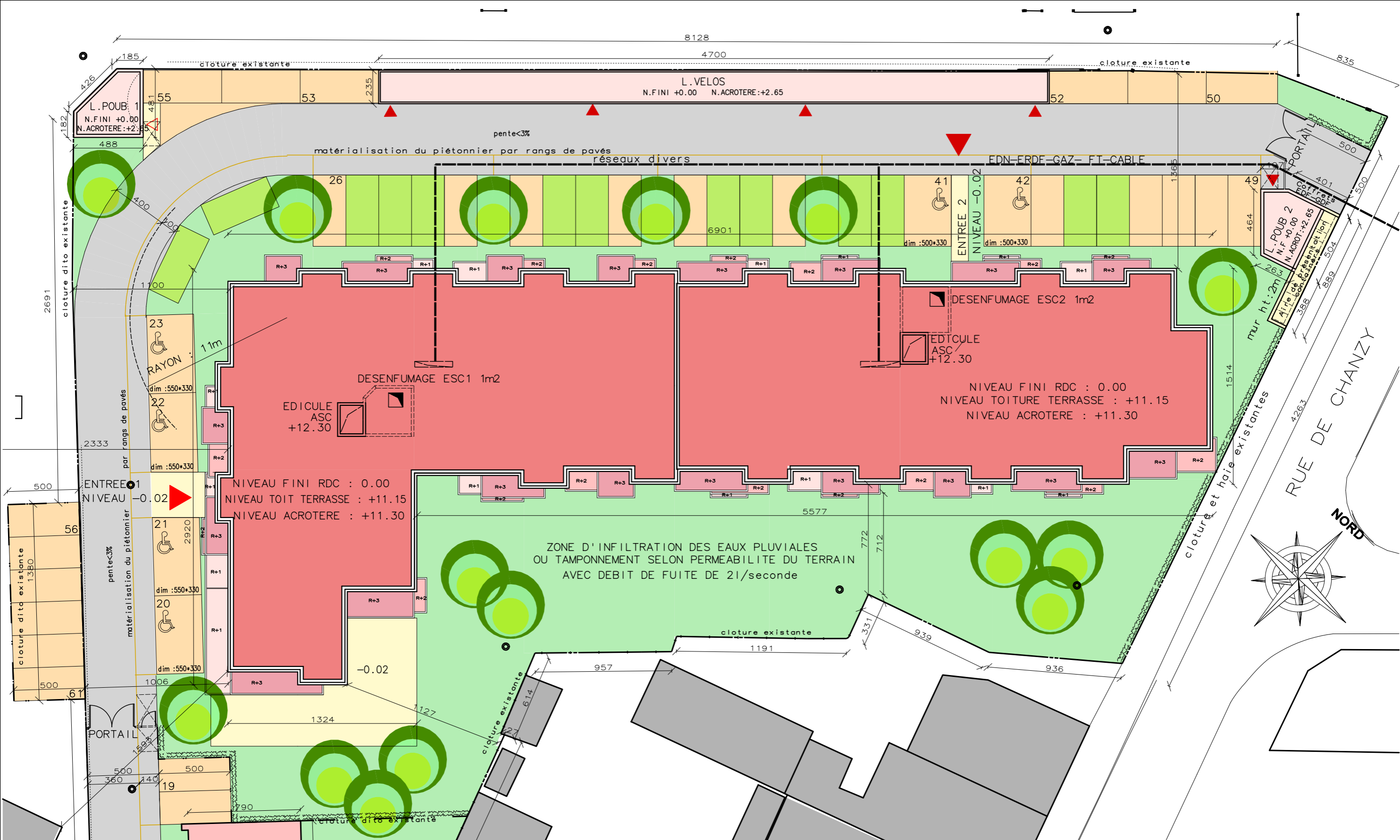
PLAN DE MASSE : Zone clôturée
