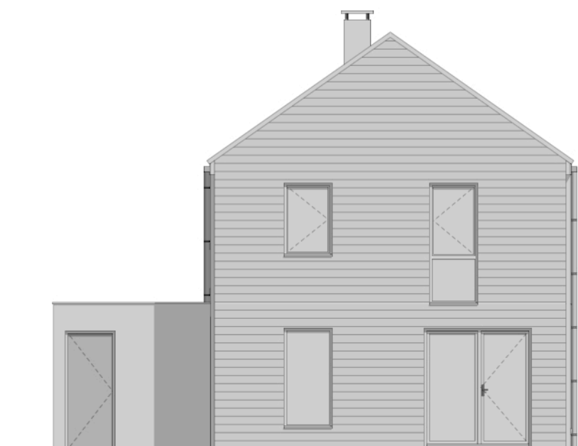
N°6 T4 Façade jardin 1:100
