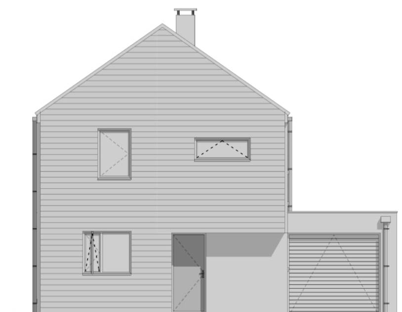
N°6 T4 Façade rue 1:100
