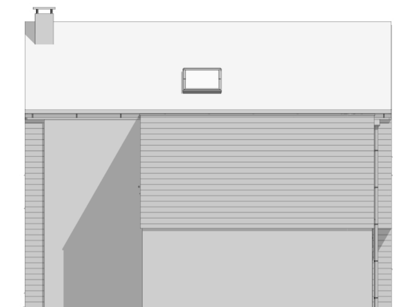
N°11 T5 Façade latérale garage 1:100
