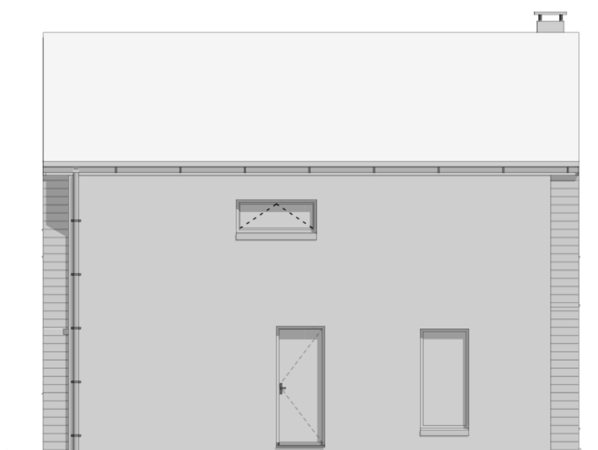
N°11 T5 Façade latérale 1:100
